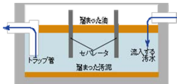
グリーストラップ断面図
