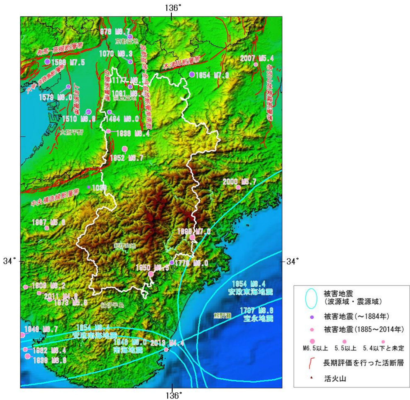
奈良県とその周辺の活断層と被害地震（地震調査研究推進本部）
