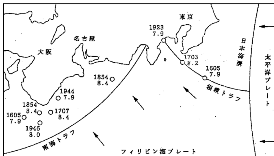
(1600 年以降、年の下の数値はマグニチュード) 相模トラフ、南海トラフと関連する巨大地震
