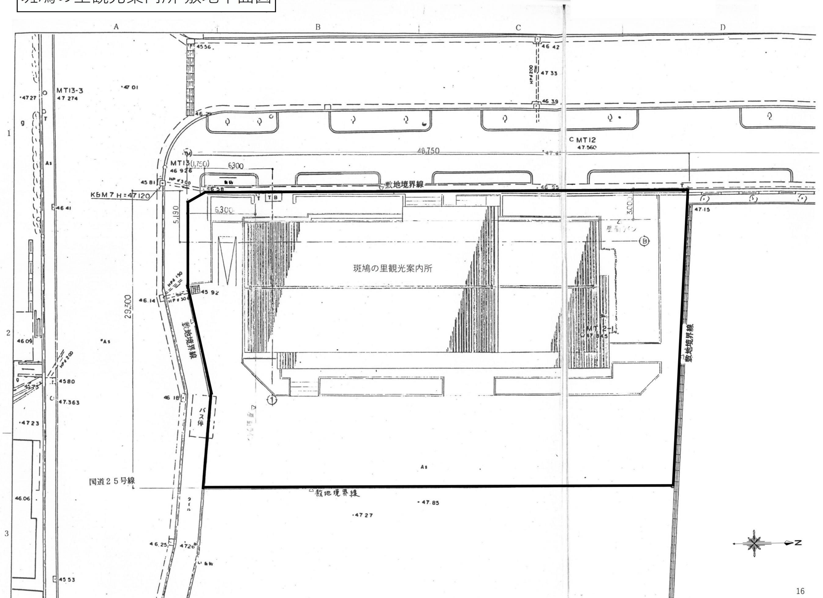
斑鳩の里観光案内所 敷地平面図
